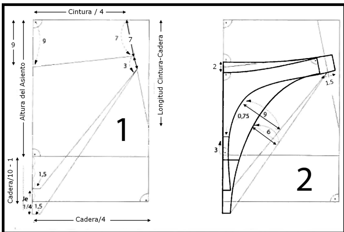
Patrón de Tanga/Colaless (2) obtenido a partir del patrón básico de Biquini (1).
